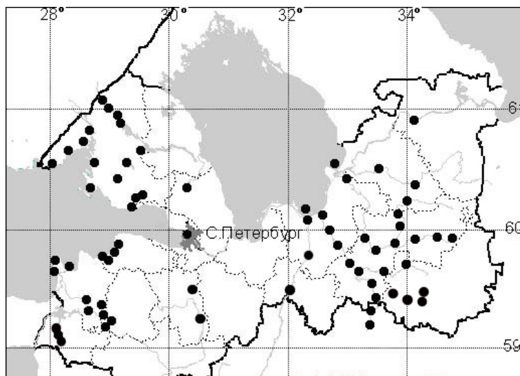
Рис. 1. Изучавшиеся водотоки Ленинградской области
