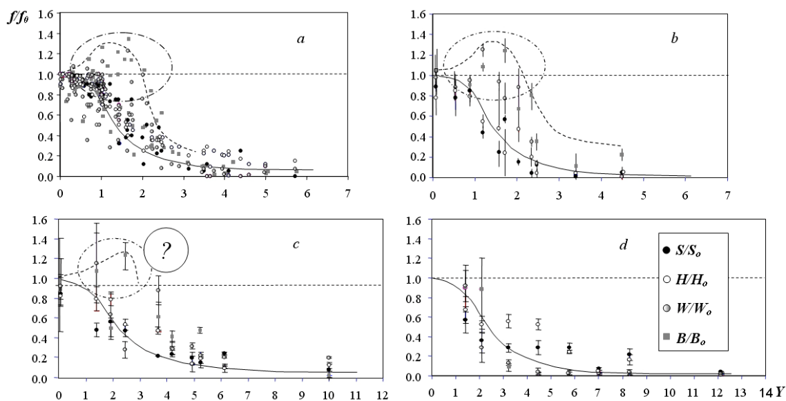
Рис. 2. Реакция макрозообентоса некоторых рек Ленинградской области на антропогенные воздействия: эвтрофирование без токсификации ( a , b ), со слабой ( c ) и со значительной ( d ) токсификацией.
